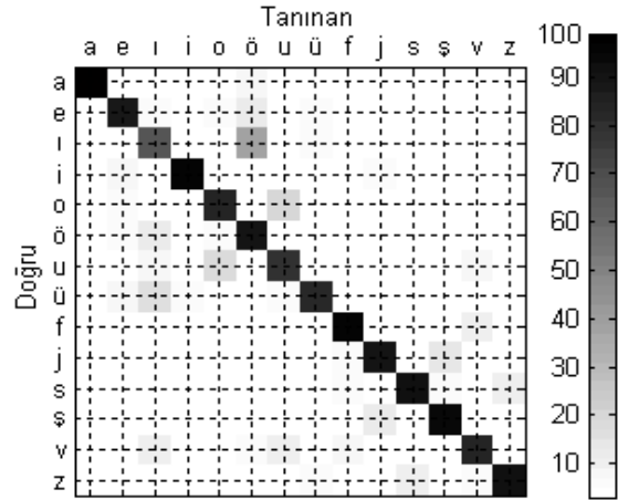
Şekil 2: Fonem tanıma oranları (%).
